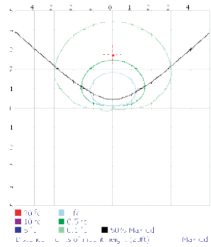
Isofootcandle Plot
