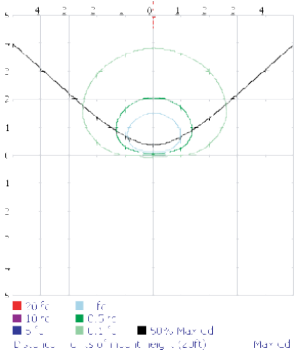
Isofootcandle Plot
